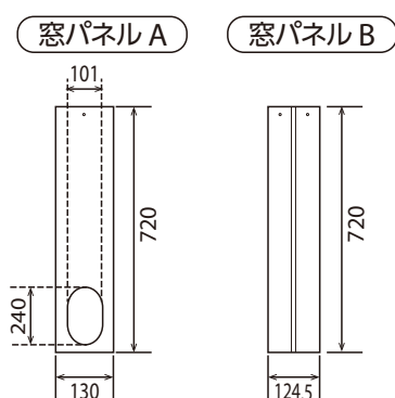
窓パネル単体寸法
