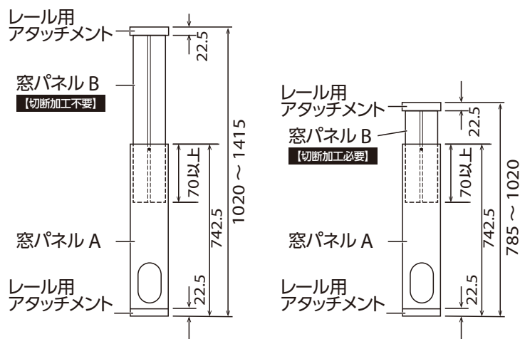
窓パネルセット寸法
