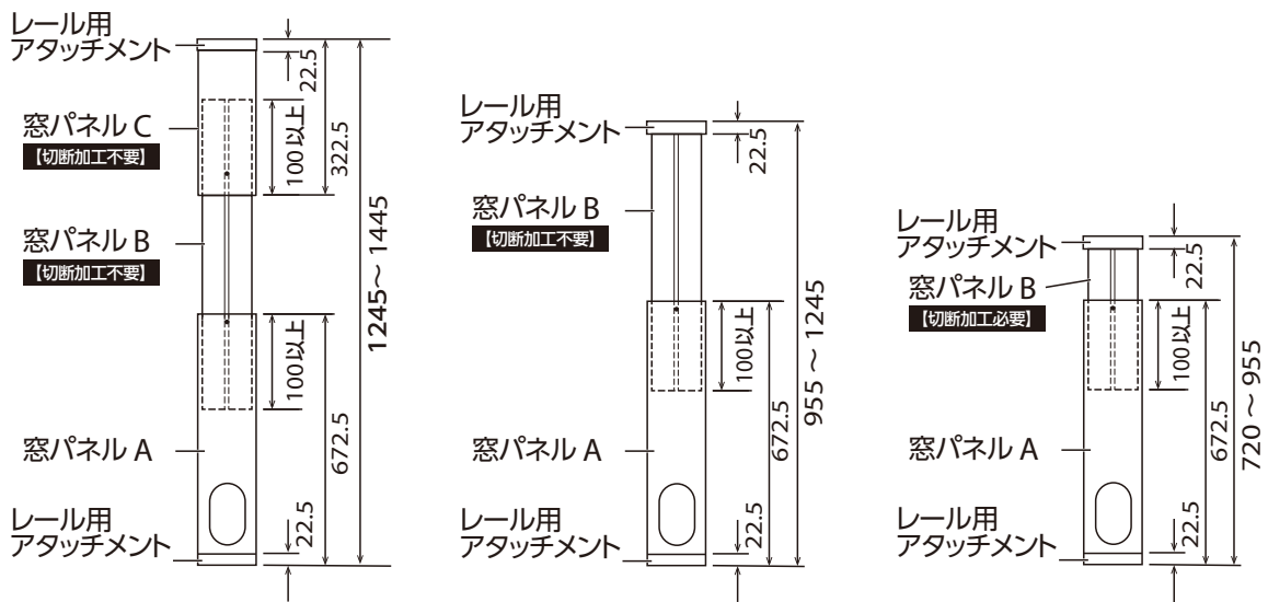
窓パネルセット寸法 ※単位mm
